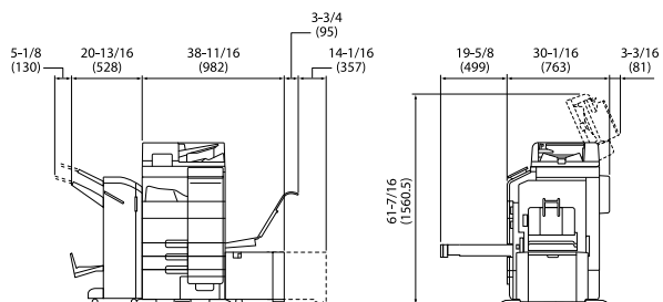
Основной блок + FS-539 SD + LU-303 + MK-730 + CU-102
